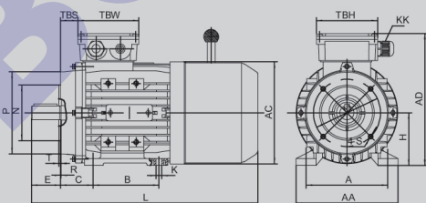
DIMENSIONES MOTORES BRIDA B34
