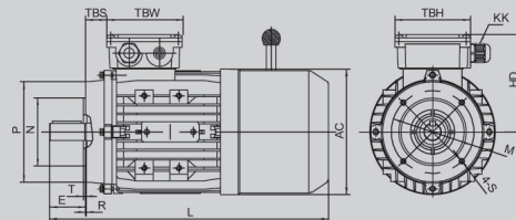
DIMENSIONES MOTORES BRIDA B14
