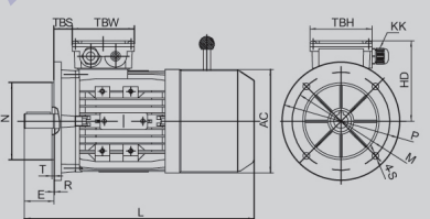
DIMENSIONES MOTORES BRIDA B5
