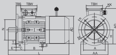
DIMENSIONES MOTORES BRIDA B35
